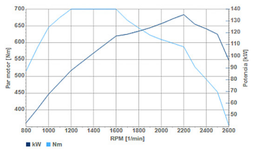
Curvas de desempeño: Motor OM 924 LA Euro V Potencia 190 cv a 2200 rpm / Torque 700 Nm @ 1200 a 1600 rpm
